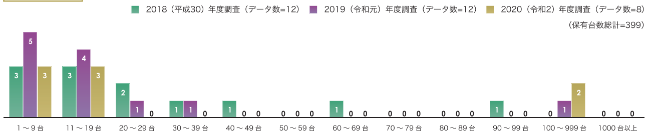
グラフ16-147 さく岩機 (ビッグハンマ)
