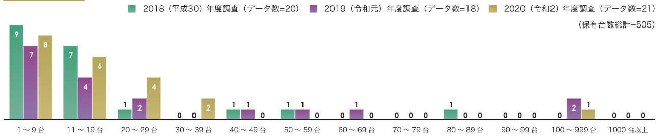
グラフ16-146 さく岩機 (レッグハンマ)
