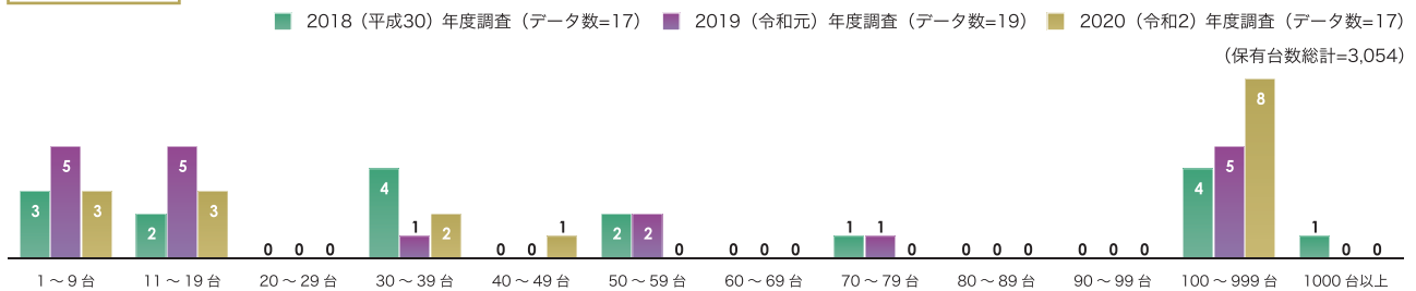
グラフ16-149 さく岩機 (大型ブレーカ)
